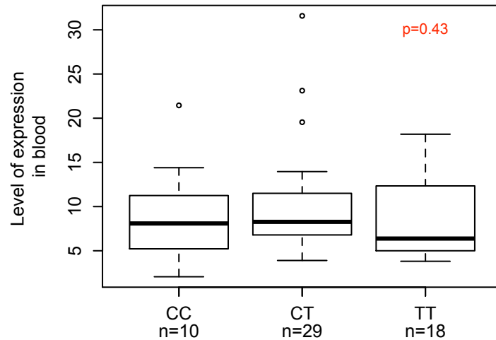
GPX4
