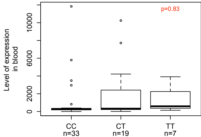
GPX1
