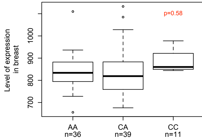
BRCA2
