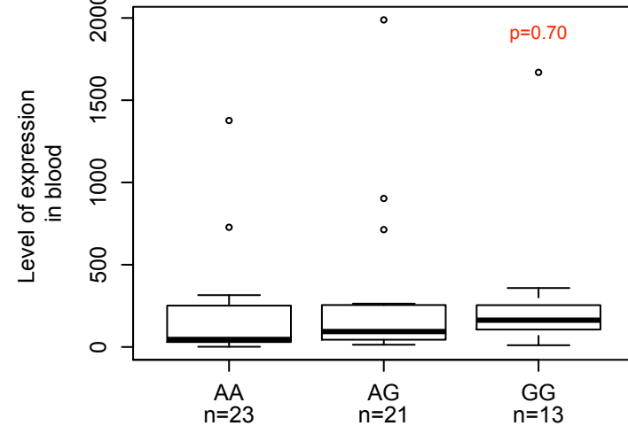
C1qA
