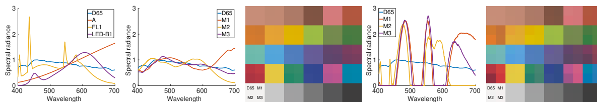
(a) 4 CIE illuminants (b) SPD of metamers (c) ColorChart of (b) (d) SPDs for max \Delta E (e) ColorChart of (d)
